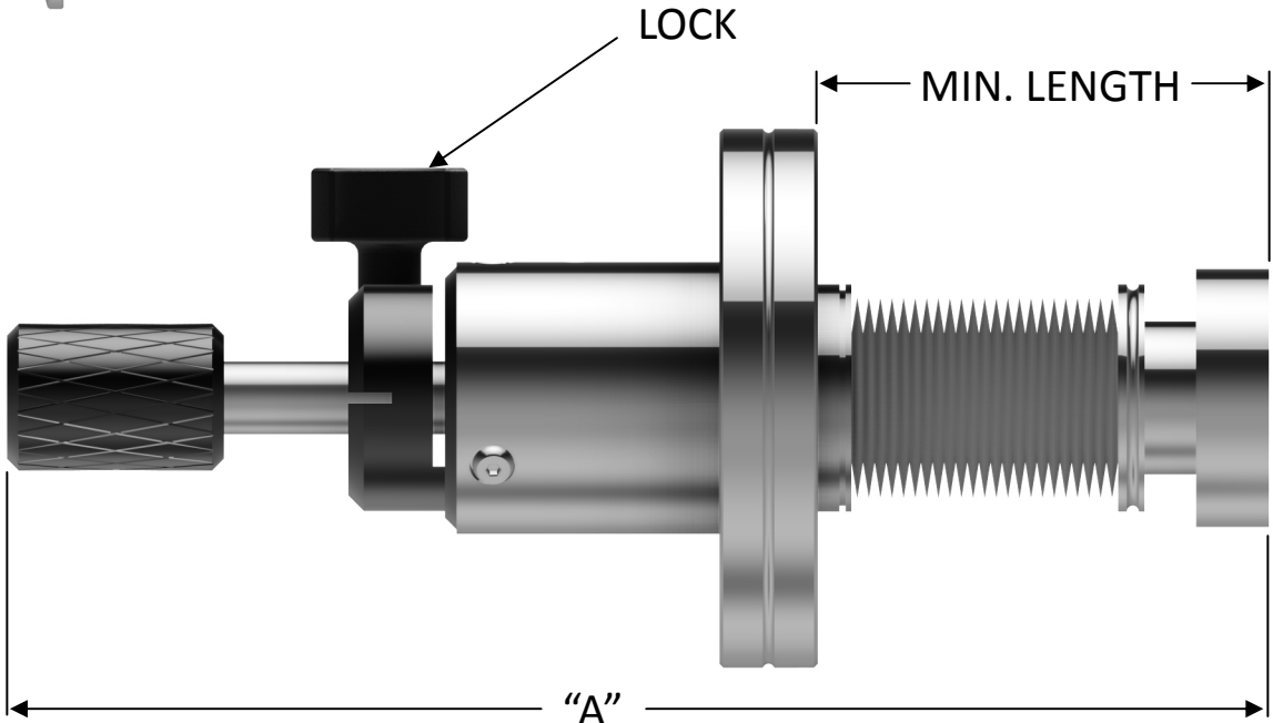
KF 40 ISO-KF
